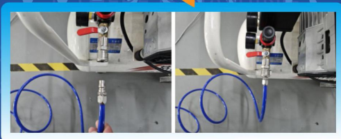
第四步：将风管快速接头对准空压机快速接头母座进行连接
